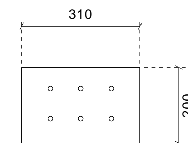
PLACA3 (e = 12.0 mm) Escala 1:10
